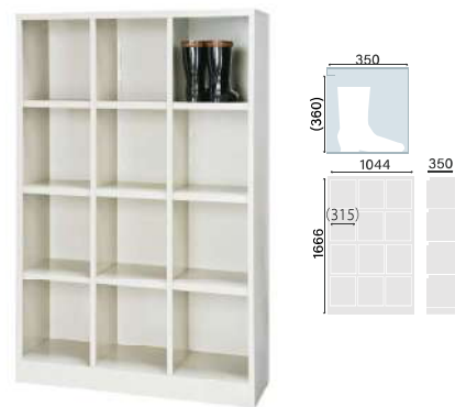
SB-2 ¥16,500 (税込) W1044×D350×H1666mm
