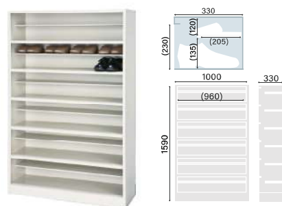
MKS-18L ¥16,500 (税込) W1000×D330×H1590mm
