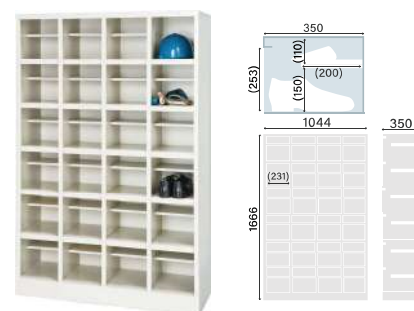
SB-1 ¥20,900 (税込) W1044×D350×H1666mm
